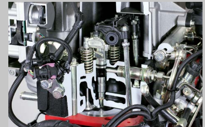
DCR Technologie. 2.000 bar Einspritzdruck garantiert maximale Motoreffizienz.
