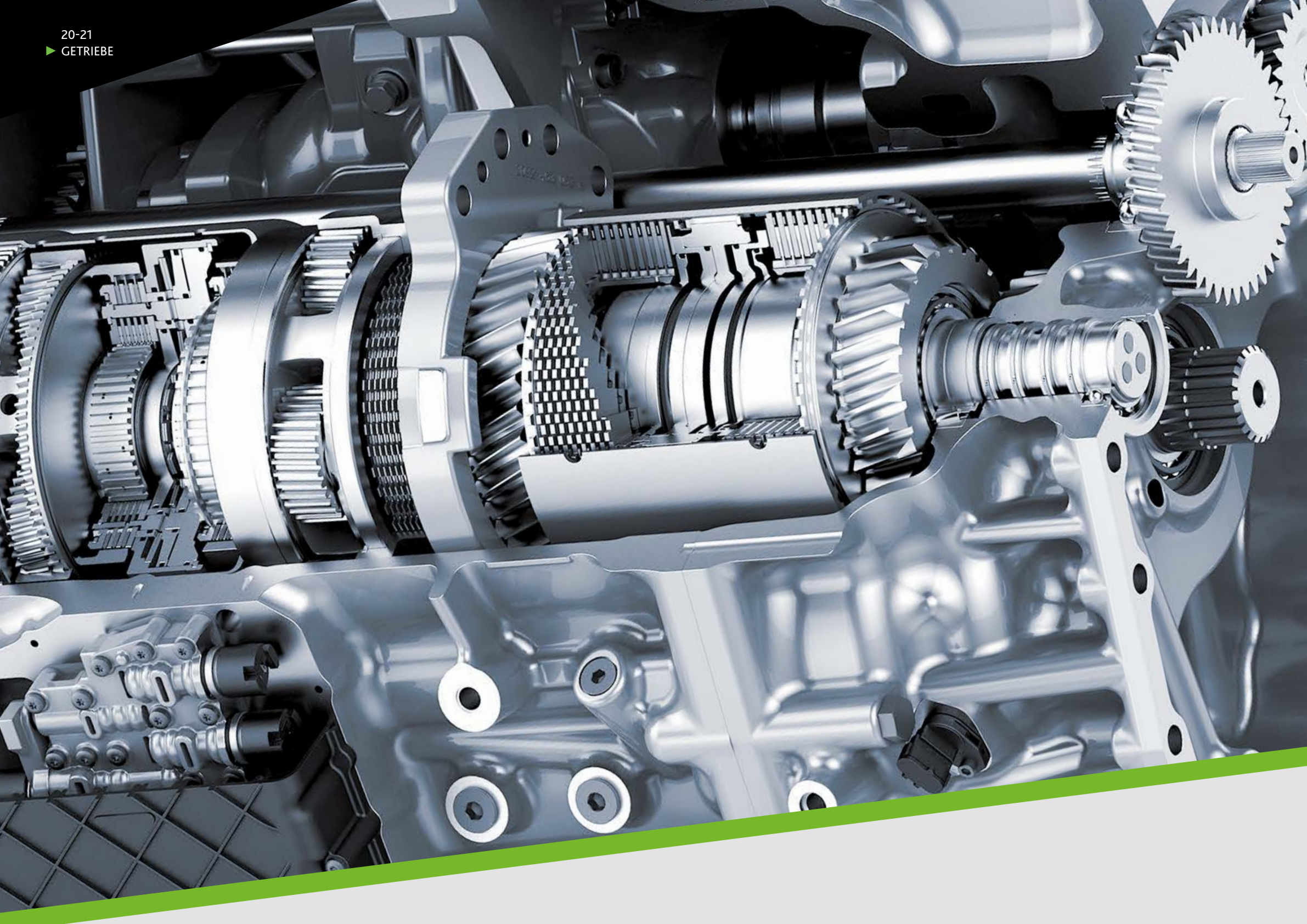
Serienmäßig: Hydraulisches Powershuttle System. Die Empfindlichkeit (Hard-Medium-Soft) wird einfach mit dem Daumen eingestellt.
