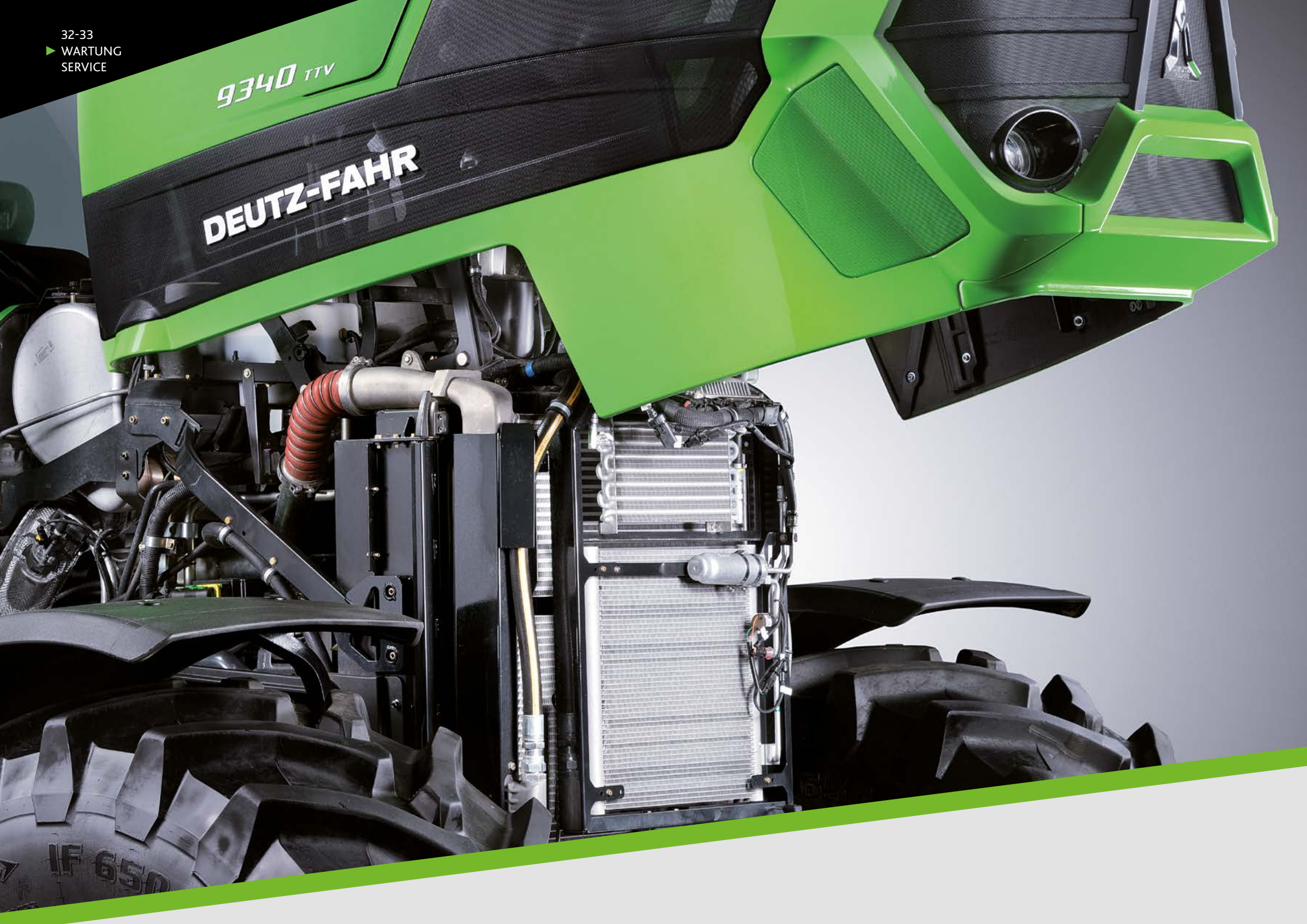
Der Kabinenluftfilter in der Kabinensäule ist einfach und werkzeuglos zugänglich.
