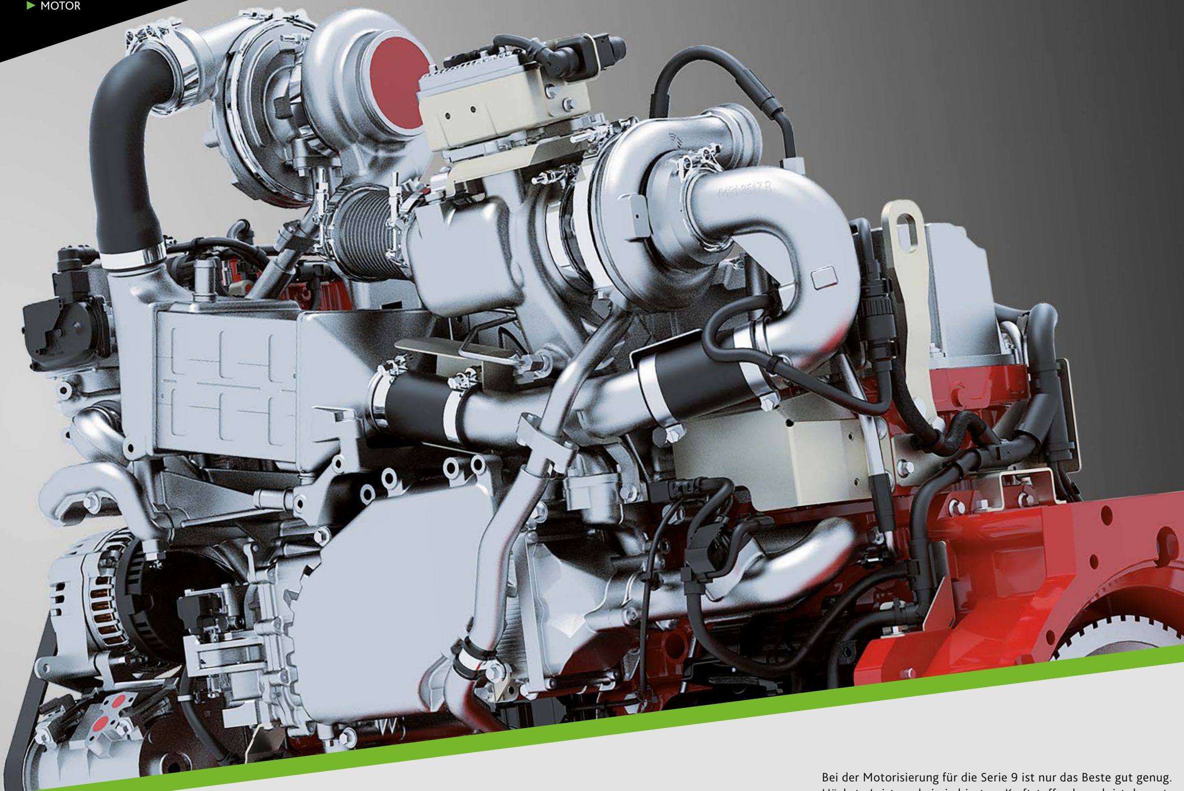
Das kompakte Kühlsystem unterstützt die Motoreffizienz und ist leicht zu warten.
