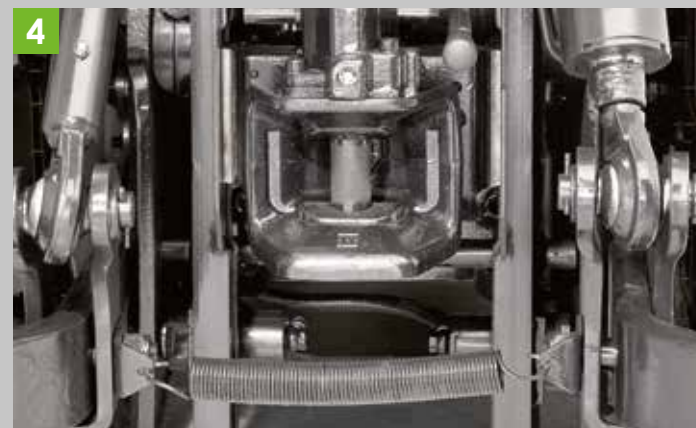
Seitenstabilisator, hydraulische Hubstrebe, Anhängerkupplungen, zur Ergänzung des Heckanbauraumes.
