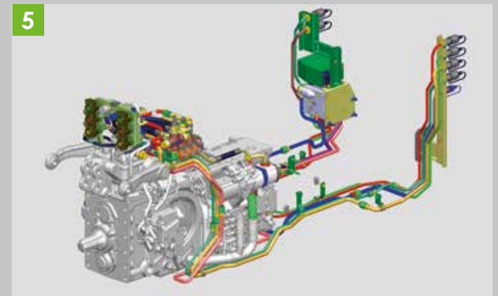
Fünf fest definierte Hydraulikpakete von einfach bis High-Tech.
