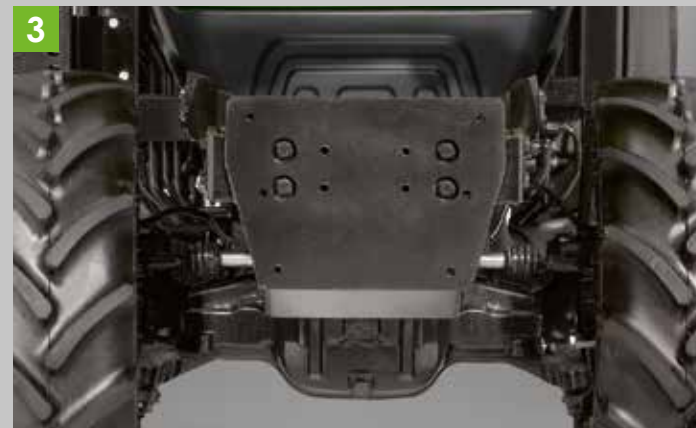
Frontanbauplatte für den schnellen und robusten Anbau von Spezialgeräten
