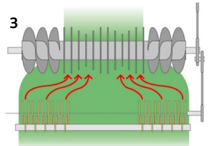
INTEGRALROTOR-Technologie
