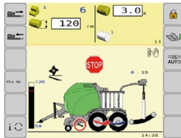
Vollautomatisches Rotor-DEBLOCK-System (nur VM BP)
