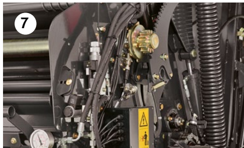
Proportionalventil für Dichteregelung von der Fahrerkabine aus
