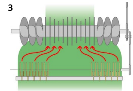
INTEGRALROTOR-Technologie
