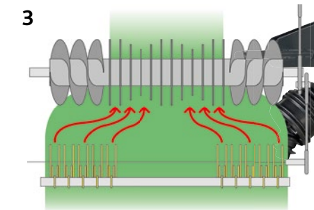
INTEGRALROTOR-Technologie
