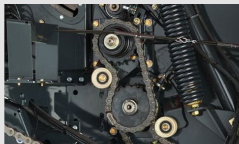
Zweiter Riemenantrieb
