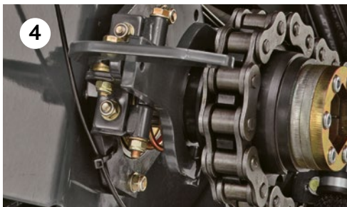
Mechanische Rotorkopplung
