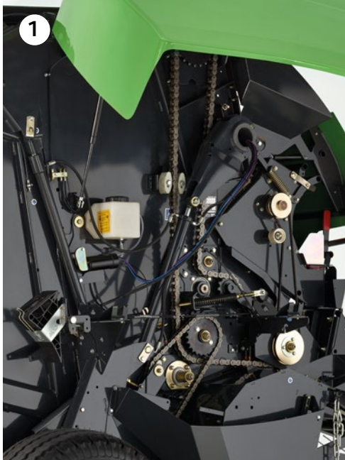
Robuster Antrieb mit hochwertigen IWIS-Ketten
